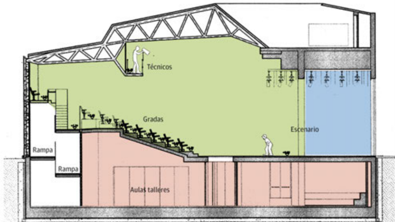
Sección. Vista lateral
