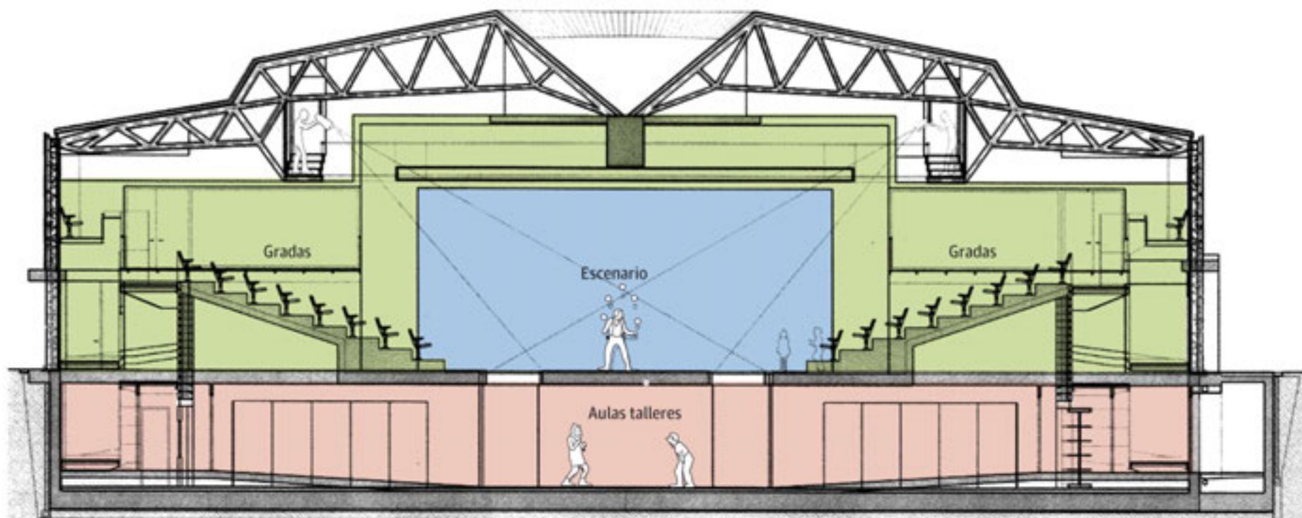
Sección. Vista frontal
